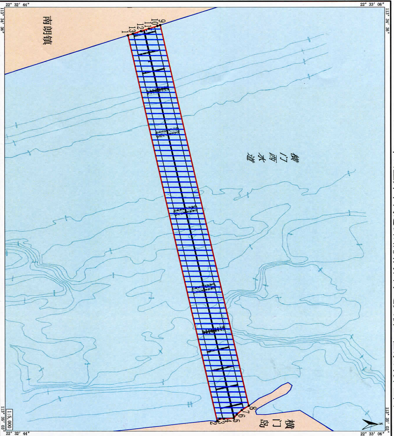
中山至开平高速公路横门西水道大桥工程宗海界址图
