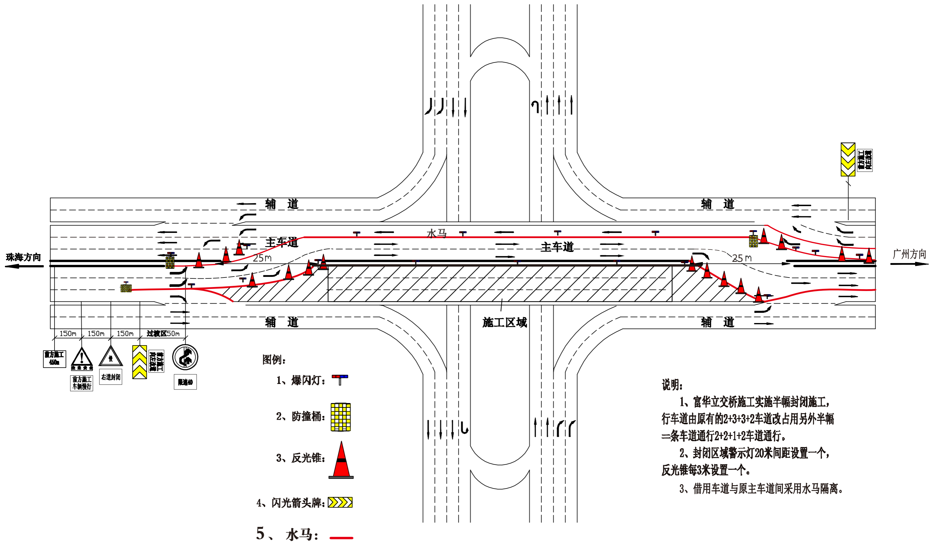
富华立交桥施工改道平面布置图
