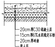
1 消防车横断面图 1:20
