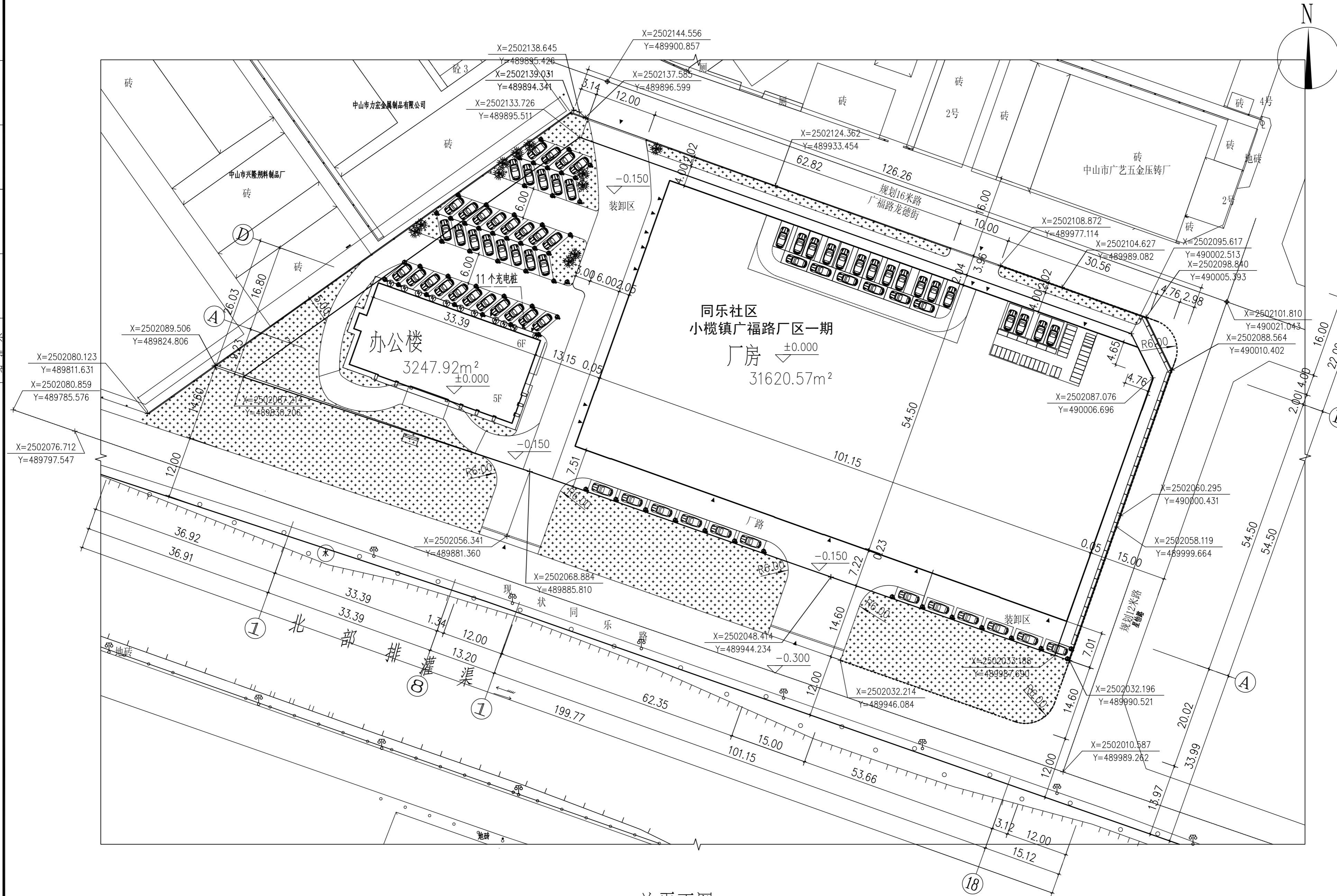
总平面图 1:500
