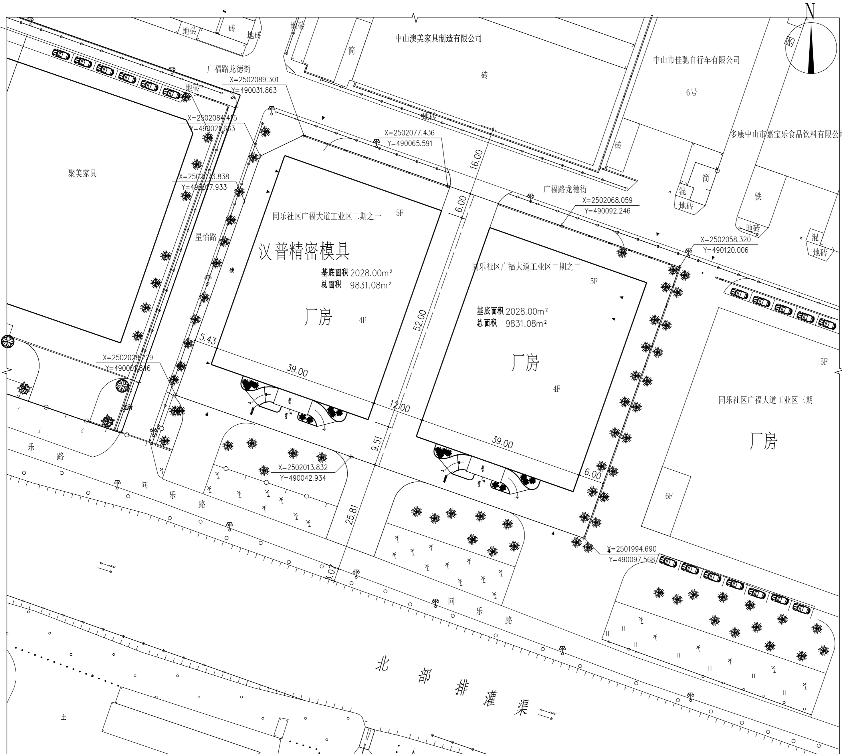
总平面图 1:500 单位:米
