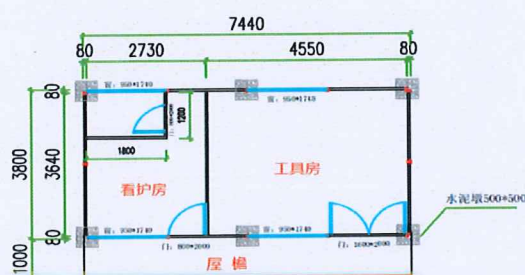
2K*4K*3P(平面图)
