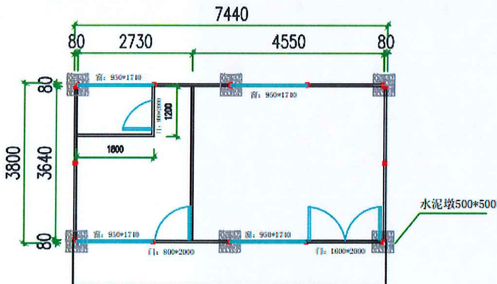
横栏镇田园看护房（工具房）样式示意图
