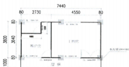
2K*4K*3P (平面图)
