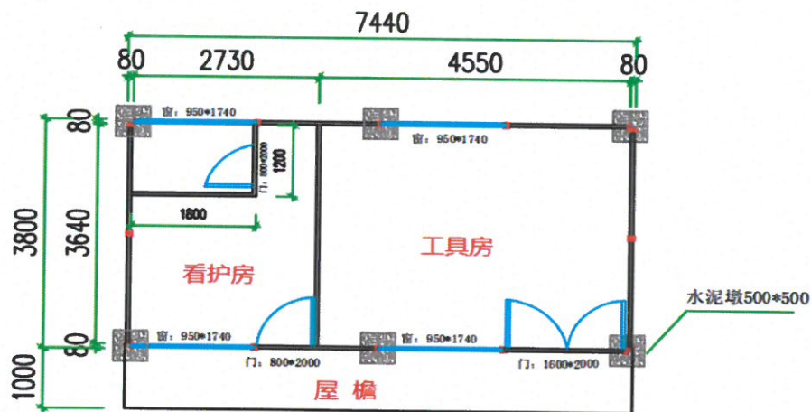
2K*4K*3P(平面图)
